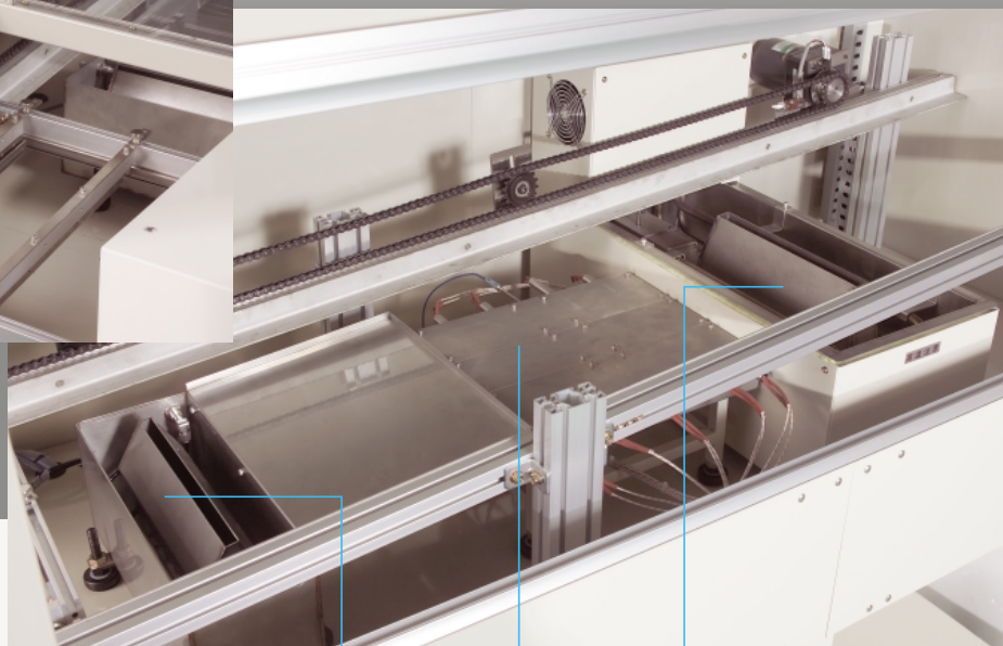
フラクサー → プレヒーター → 半田槽
